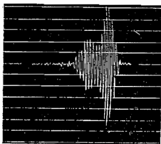
Santiago. Péndulo Bosch Omori Comporente NW-1,909-Junio 8-IV-38-8
