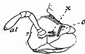
Fig. 4.—CABEZA MUI AUMENTADA DE GLOMERIS CONVEXA, mostrando en x el órgano de Tömösvary.
